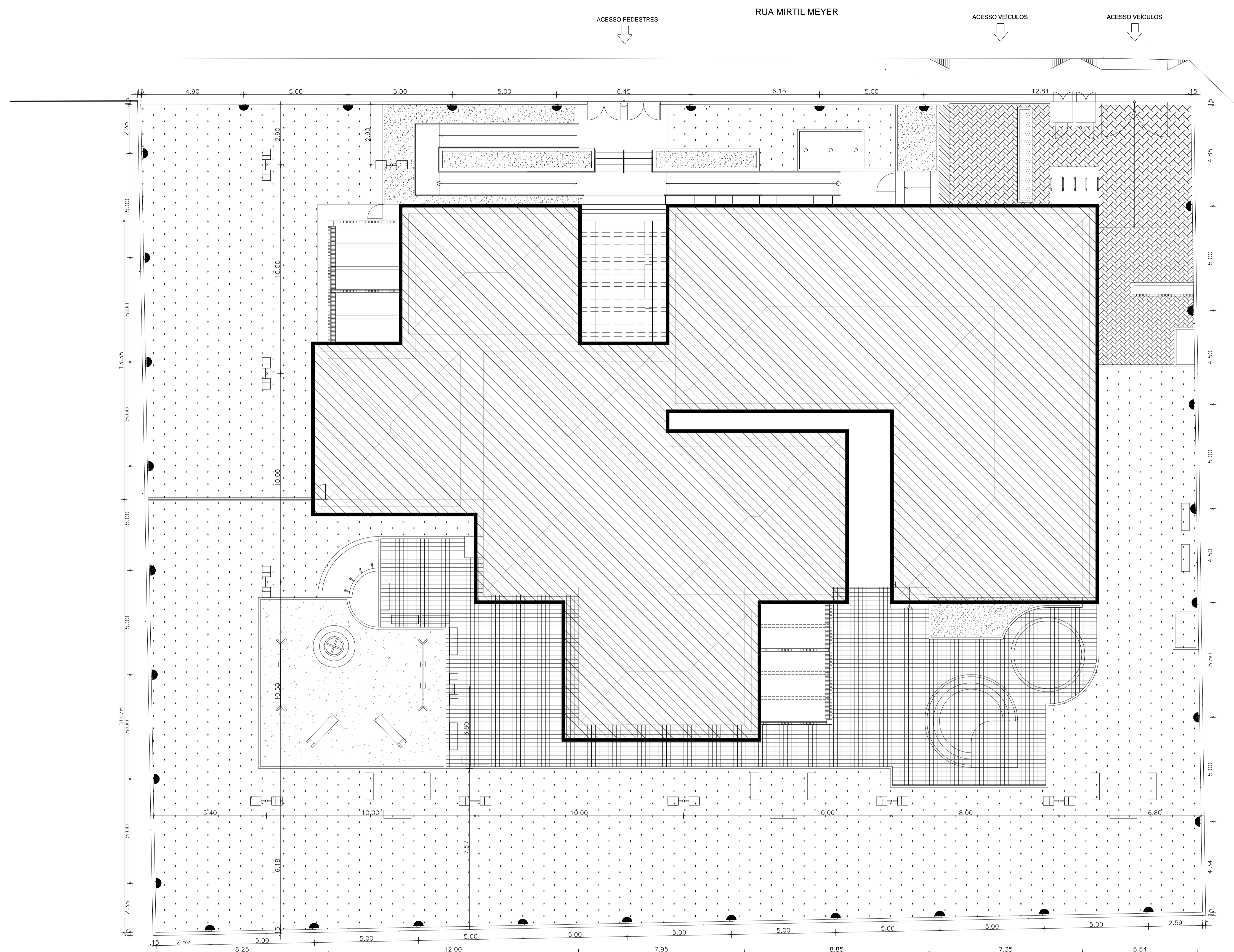
01 PLANTA DE ILUMINAÇÃO ESCALA: 1:100
